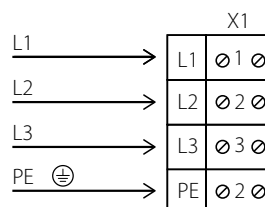
Схема подключения к электросети для вентилятора с модификацией корпуса с клеммной коробкой
