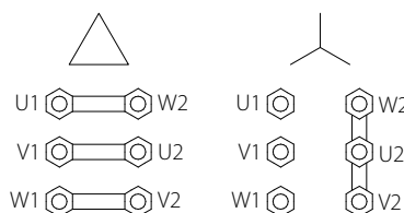
Схема подключения к электросети для вентилятора с модификацией корпуса без клеммной коробки
