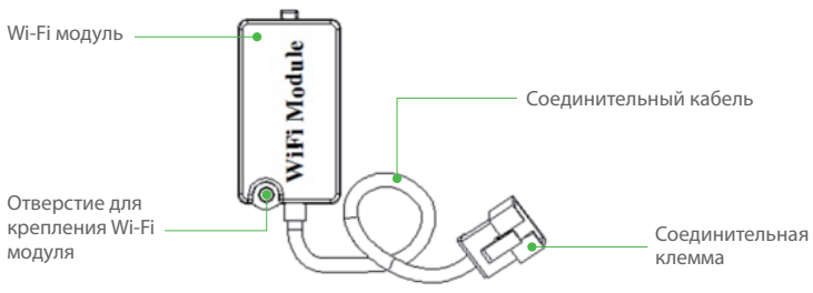
Схема Wi-Fi модуля
