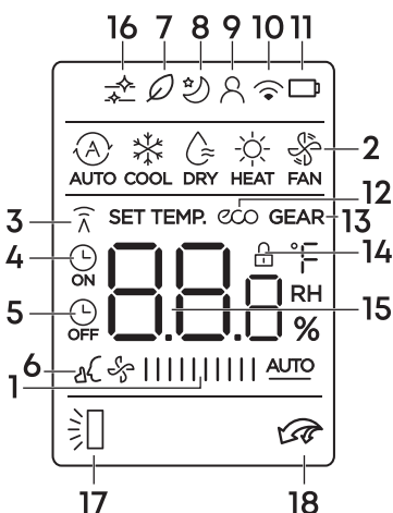
Рис. 4. Индикация на дисплее
