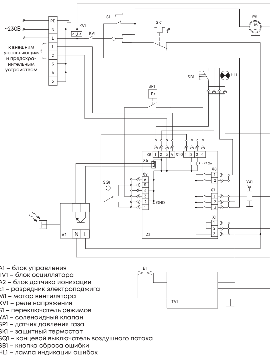
Рис.6. Электрическая принципиальная схема для воздухонагревателей BSG-33, BSG-45, BSG-70, BSG-95
