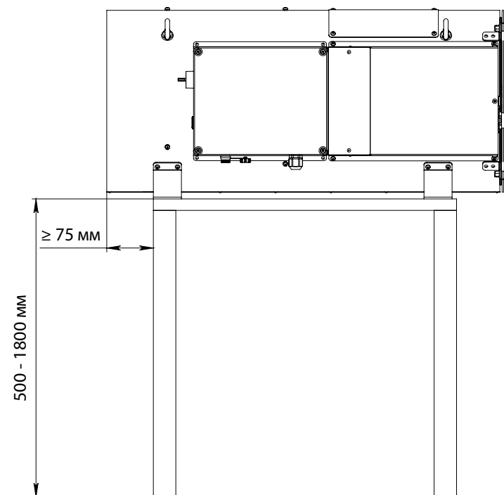
Рис. 2. Установка изделия на опорном основании
