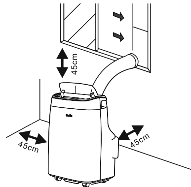
Рис. 10. Монтаж кондиционера.
