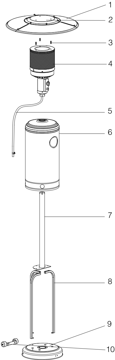
Рис. 3 – Комплектация
