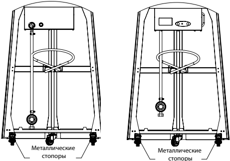
Рис. 9 Установка стопоров
