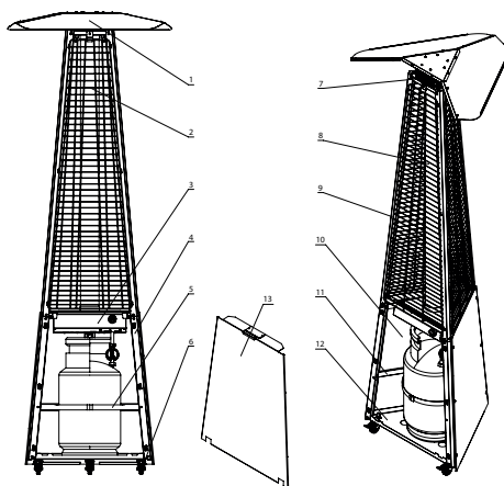
Рис. 2. Устройство модели BOGH-15
