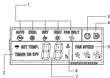
ЖК-дисплей проводного пульта управления
