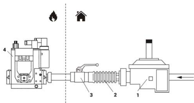
1: filtre-régulateur de pression ou filtre 2: joint anti-vibrations 3: vanne d'arrêt 4: rampe de gaz
