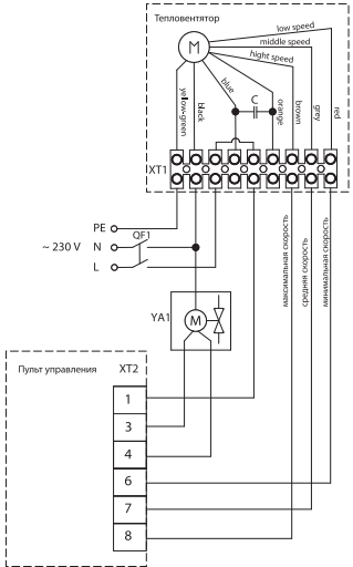
XT1 - XT2 колодка клеммная; YA1 - прибор электромагнитного вентилia; QF1 - автоматический выключатель.
