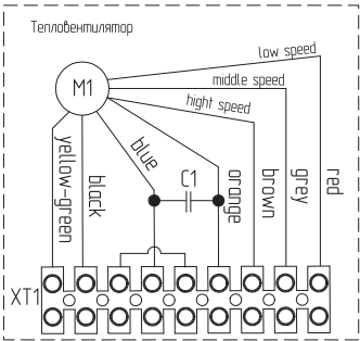
Внутренняя схема клеммной коробки тепловентилятора.
