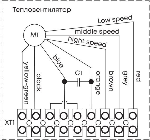
Внутренняя схема клеммной коробки тепловентиллятора.
