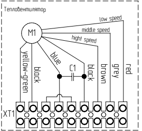
Внутреннее устройство клеммной коробки.
