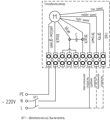
Подключение водяного тепловентилятора через автоматический выключатель.
