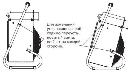
Рис. 3. Тепловентилятор
