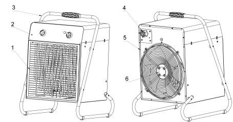
Рис. 2. Модели ВНР-М2-30
