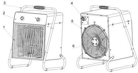
Рис. 2. Модели ВНР-М2-30
