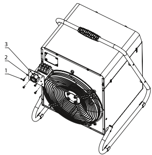
Рис. 5. Схема подключения к стационарной электросети
