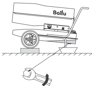
рис. 8 Опорожнение топливного бака для ВНДР-30, ВНДР-50
