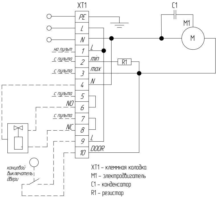
Схема электрическая принципиальная тепловых завесы ВНС-Н15W30-SP
