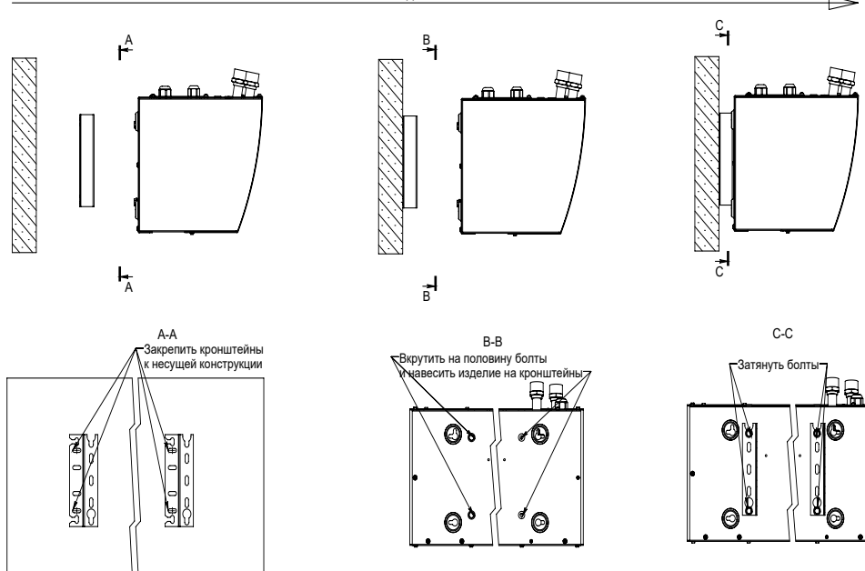
Схема крепления завесы горизонтально над проемом к стене с помощью кронштейнов ПОСЛЕДОВАТЕЛЬНОСТЬ
