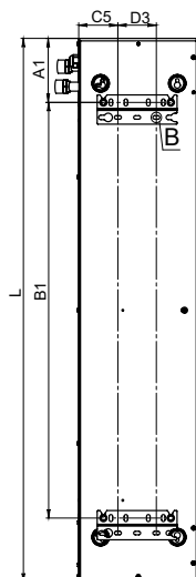
Расположение кронштейнов для вертикальной установки
