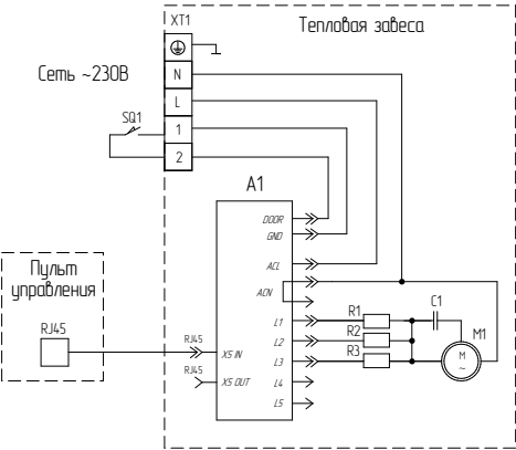
Схема электрическая принципиальная воздушной завесы ВНС-Н10А-PS:
