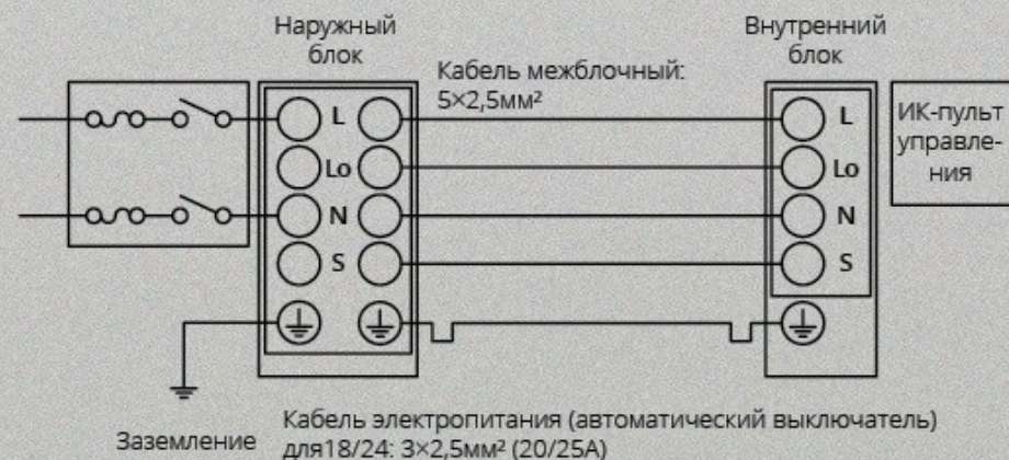
Схема подключения Q inverter (18/24)
