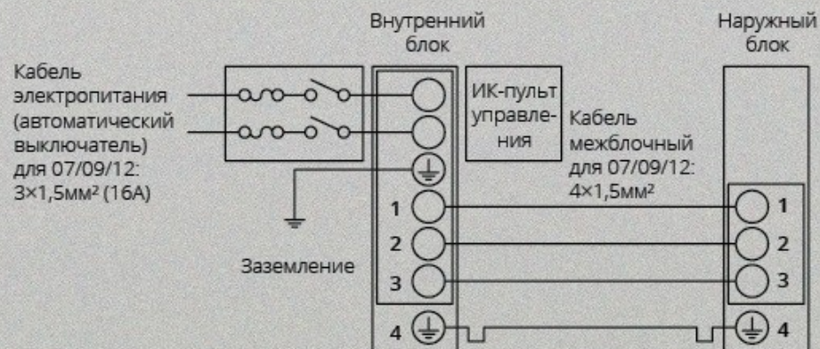
Схема подключения Q Light Inverter (7/9/12)
