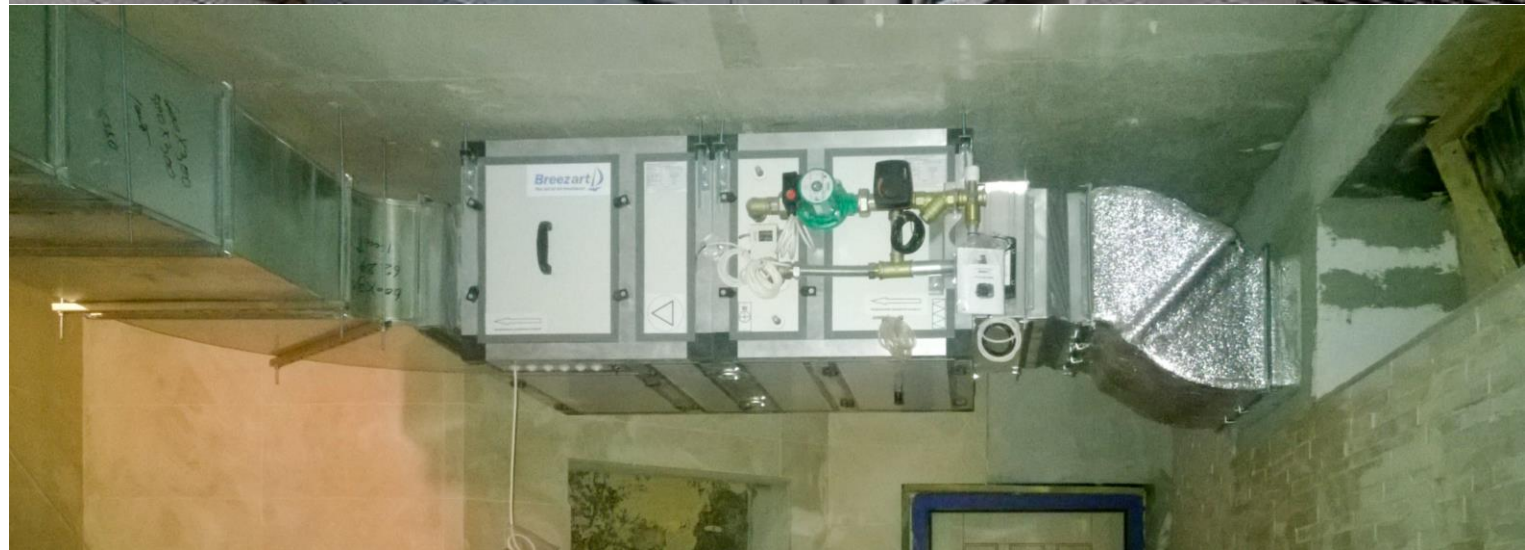
Частный дом, Московская область VRV-система Daikin, VAV-система Breezart
